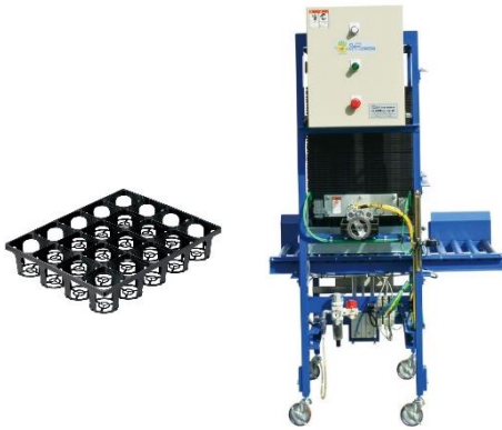
システムトレイ供給機
